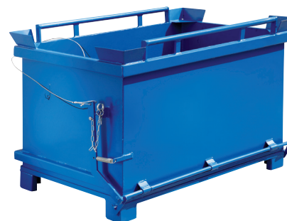
• 4727 Kontajner s výklopným dnom Objem: 1000 l Rozmery: 1500 x 1080 x 970 mm Materiál: oceľ Povrchová úprava: prášková farba
